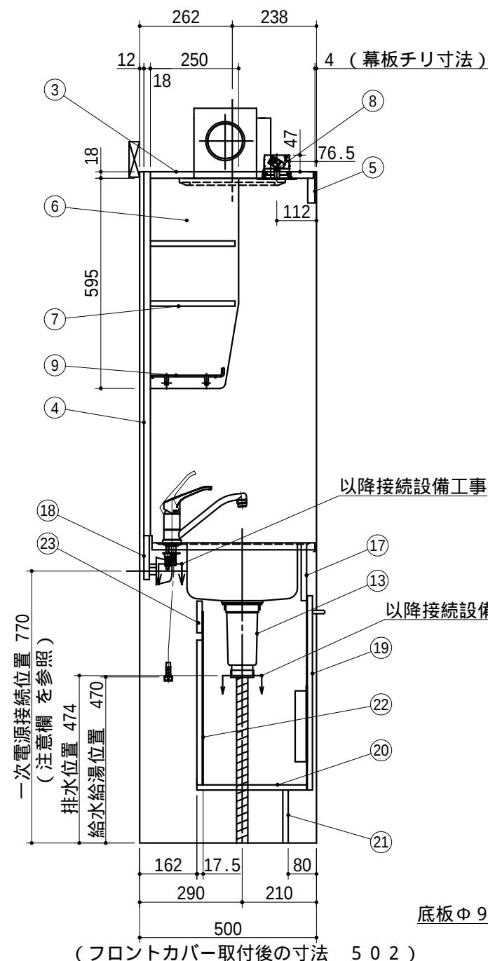
A 部詳細
