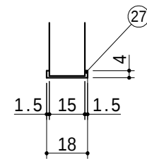
A 部詳細
