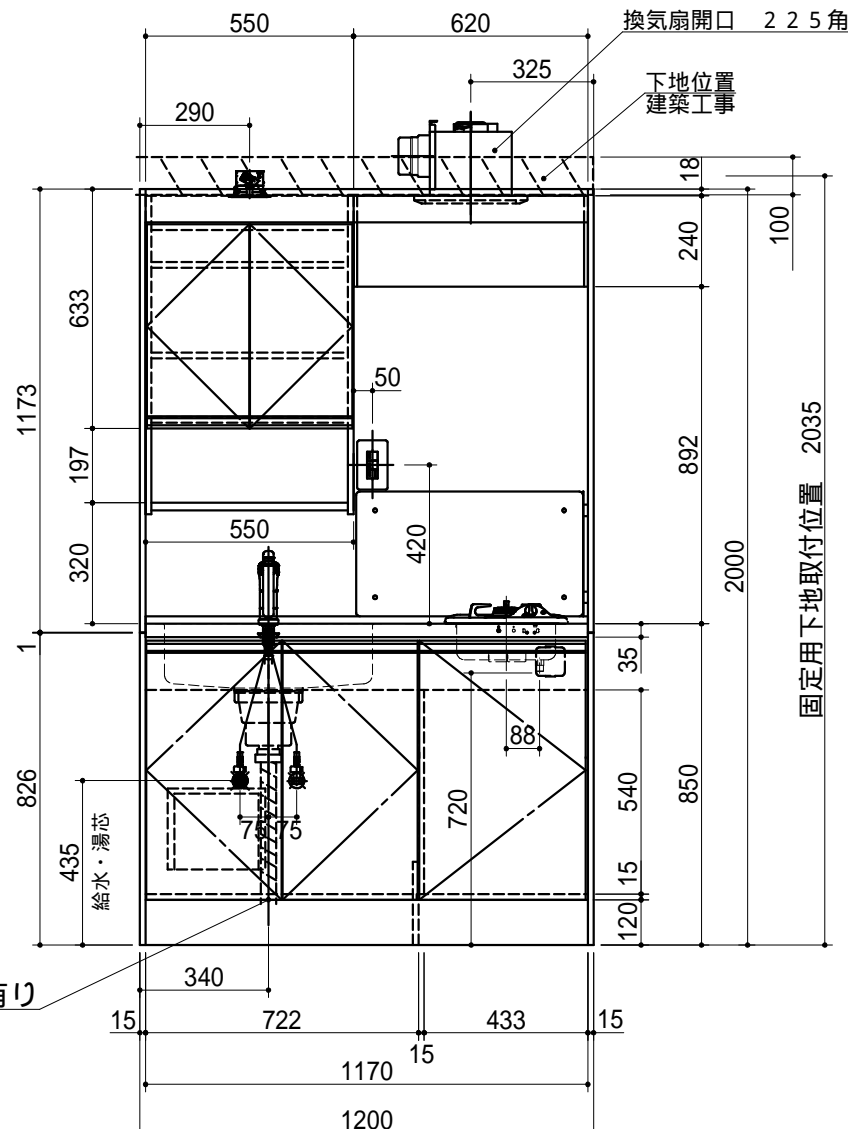
(フロントカバー取付後の寸法 1203)
