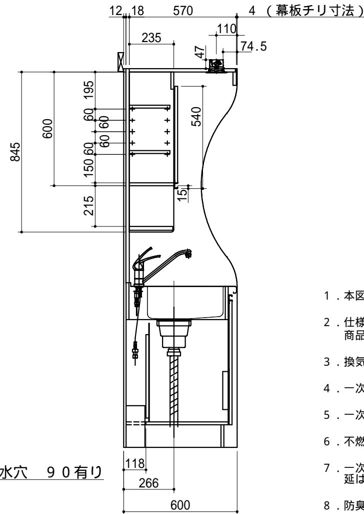
(フロントカバー取付後の寸法 602)
