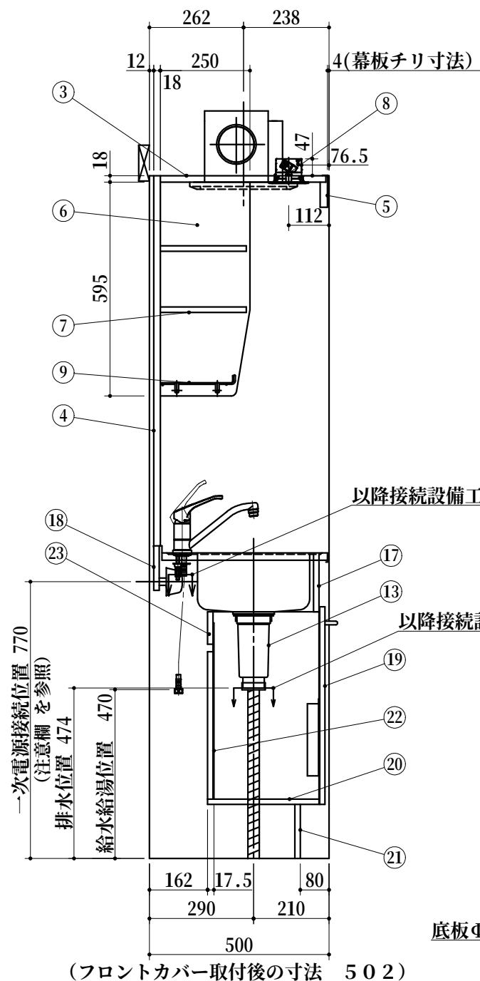
A部詳細
