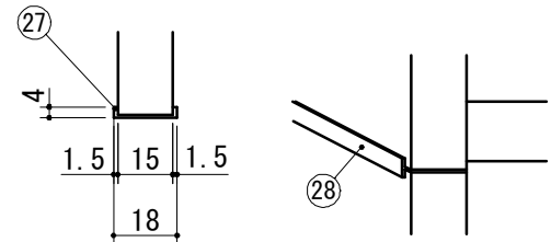
矢視B
