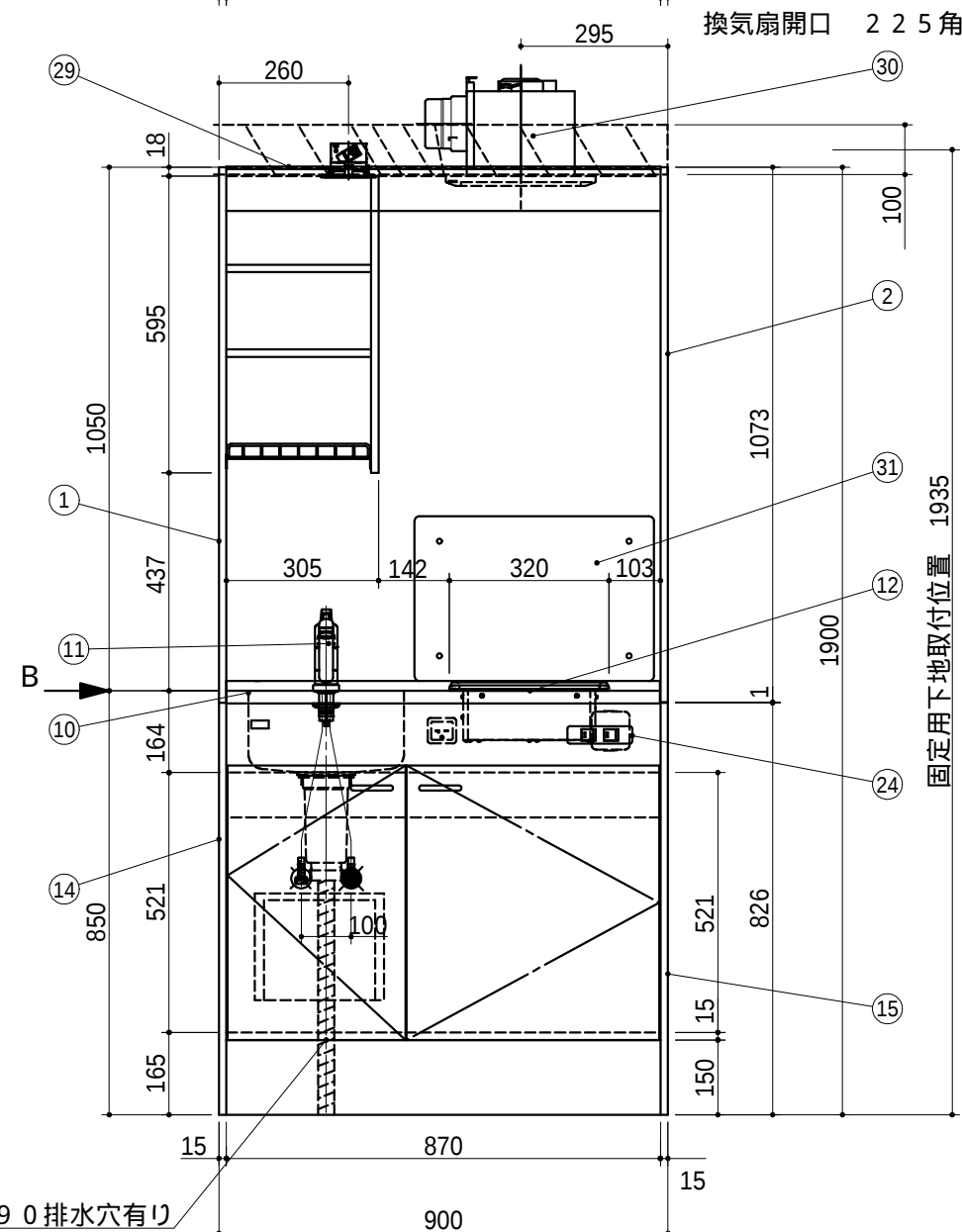
(フロントカバー取付後の寸法 903)
